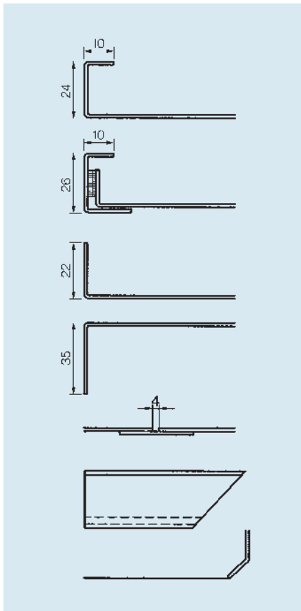
Putzanschluss P
