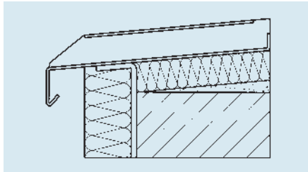
Mit Bügel ohne Isolation oder mit Isolation Montagebügel werden immer lose mitgeliefert
