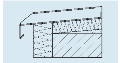
Zum Kleben ohne Isolation oder mit Isolation
