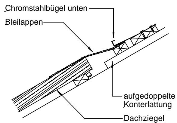
Schritt 5: Chromstahlbügel unten gemäss Rasterplan setzen. Bügel auf Bleilappen aufliegend.
