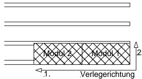
Schritt 6: Module einsetzen. Rechts beginnen und Module immer gleich nach einklinken verdrahten.
